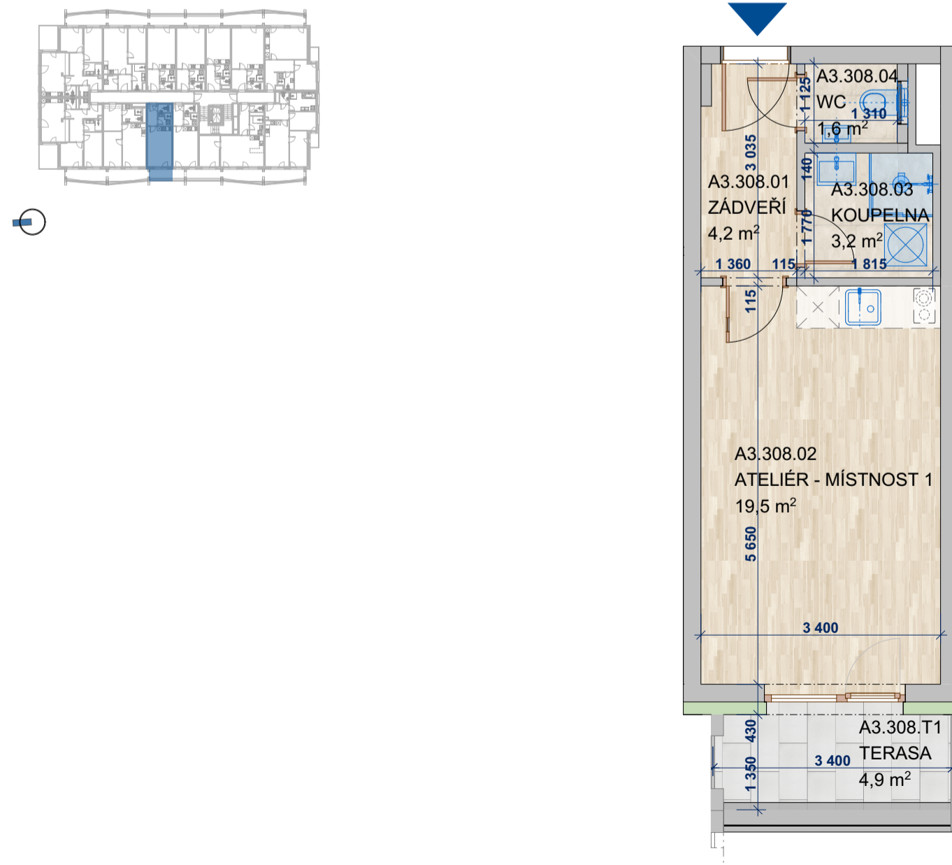
SCHÉMA PODLAŽÍ
