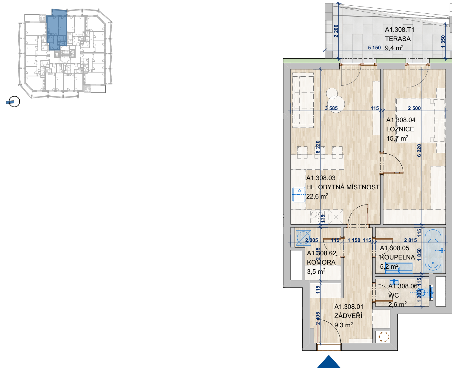
SCHÉMA PODLAŽÍ
