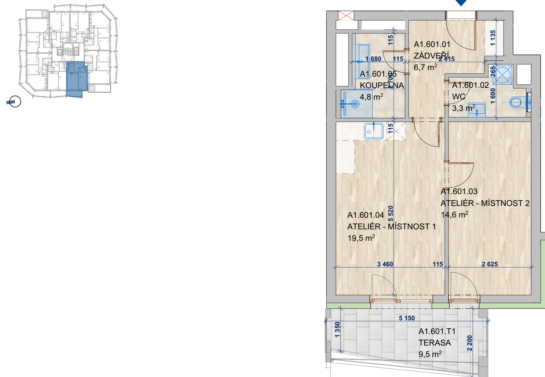
SCHÉMA PODLAŽÍ
