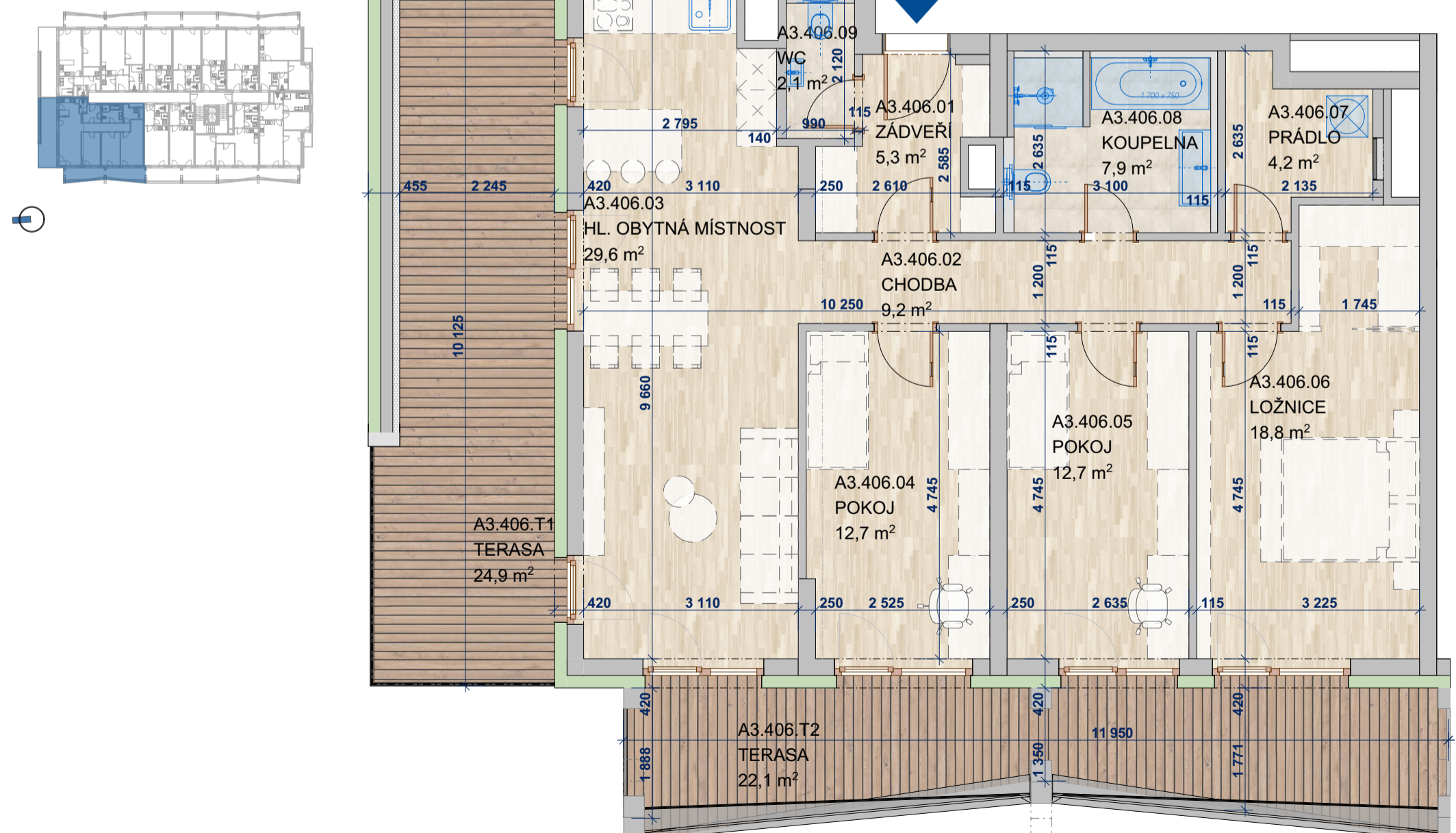
SCHÉMA PODLAŽÍ
