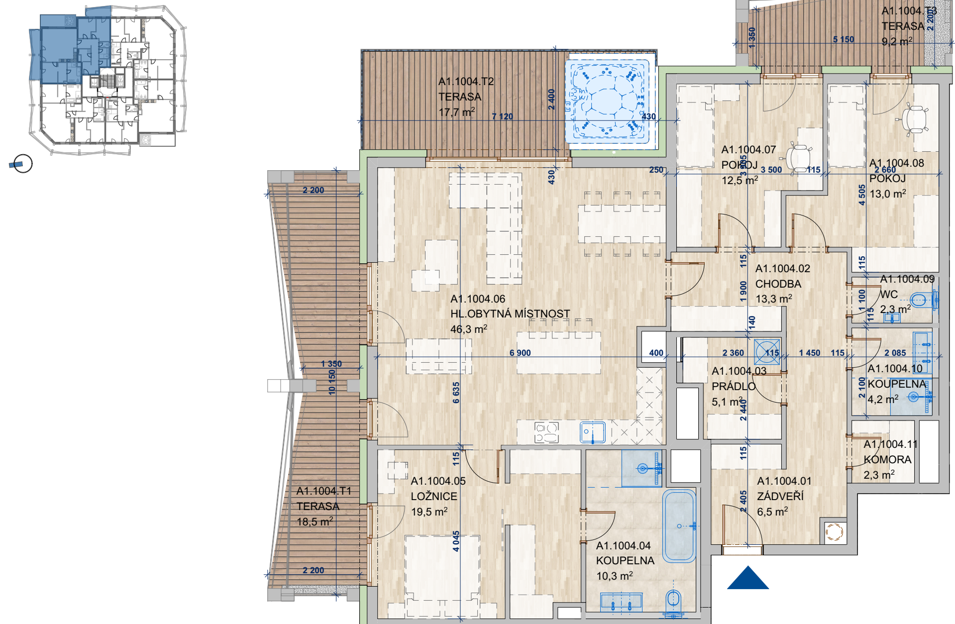
SCHÉMA PODLAŽÍ
