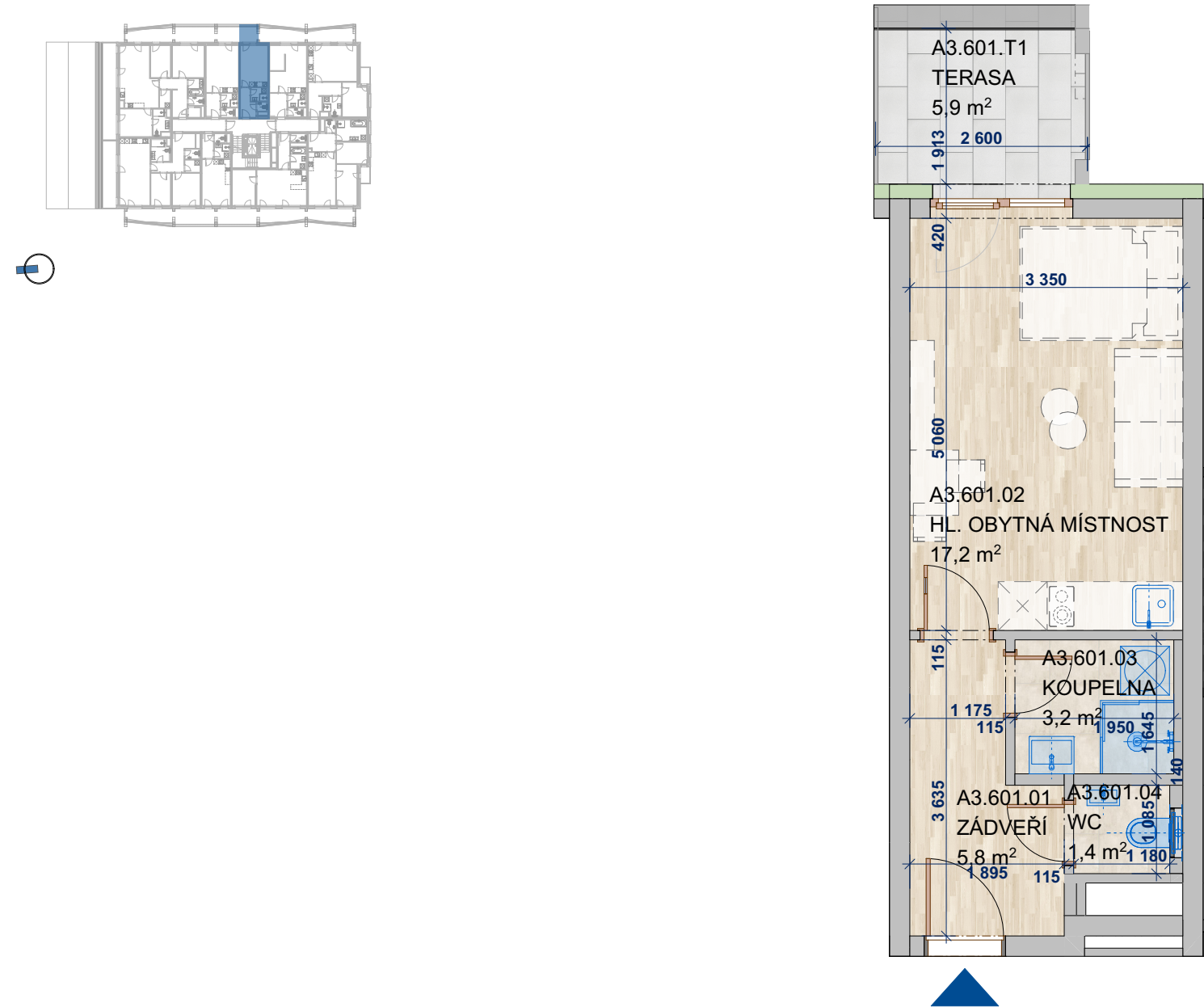
SCHÉMA PODLAŽÍ
