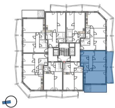
SCHÉMA PODLAŽÍ
