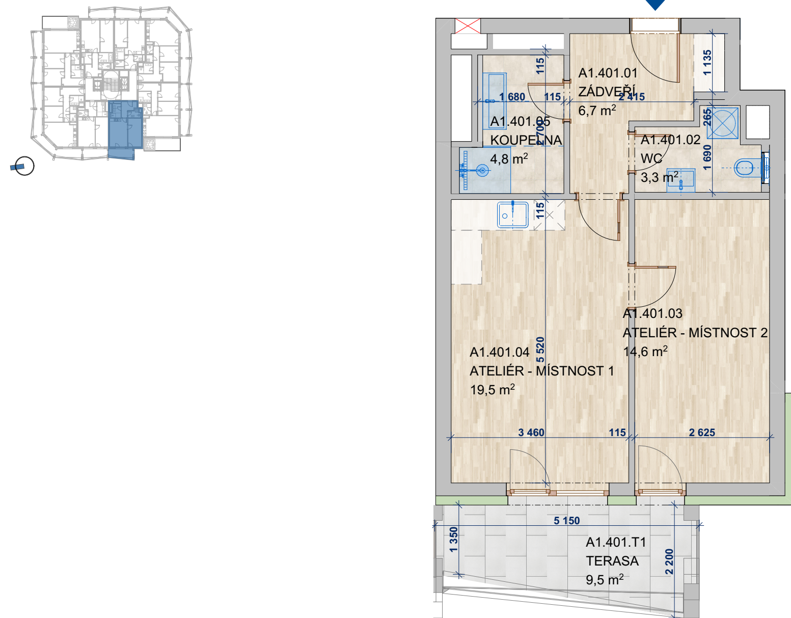
SCHÉMA PODLAŽÍ
