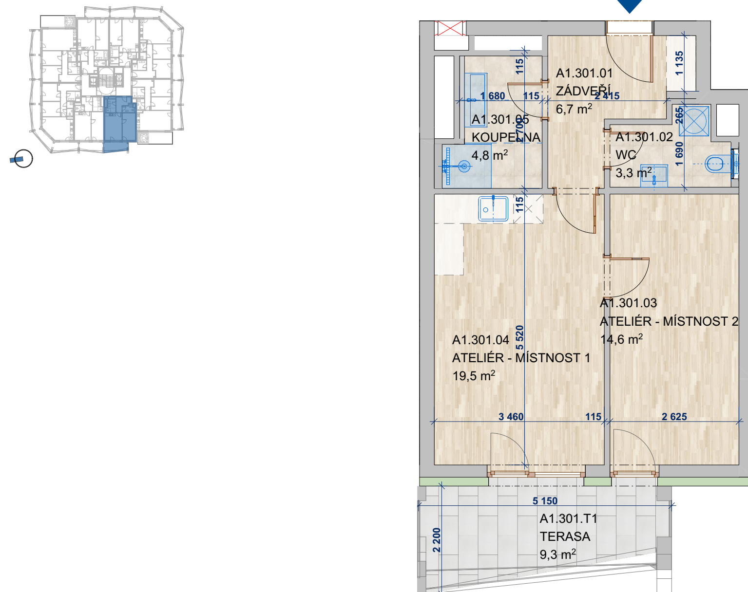
SCHÉMA PODLAŽÍ
