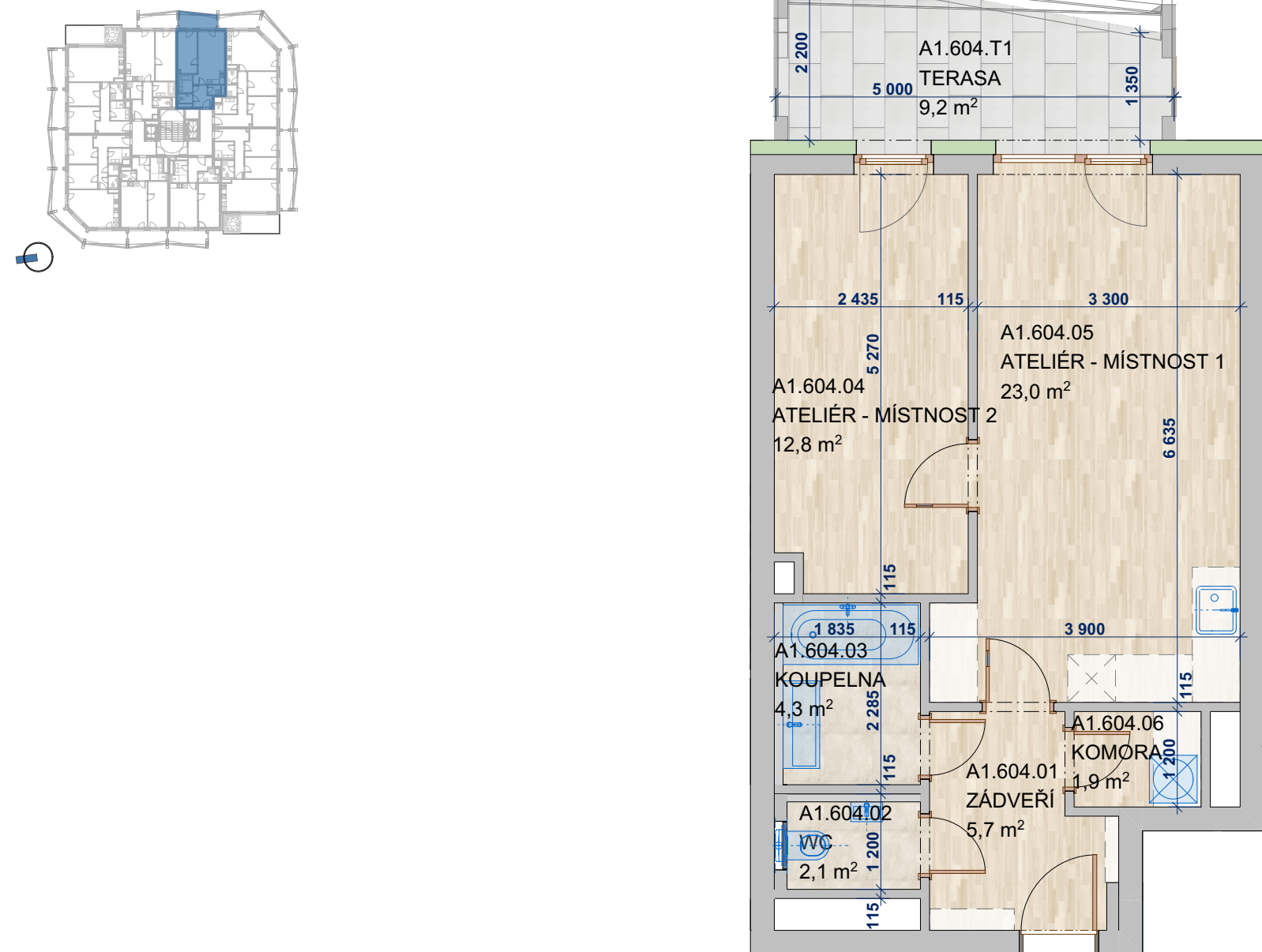
SCHÉMA PODLAŽÍ
