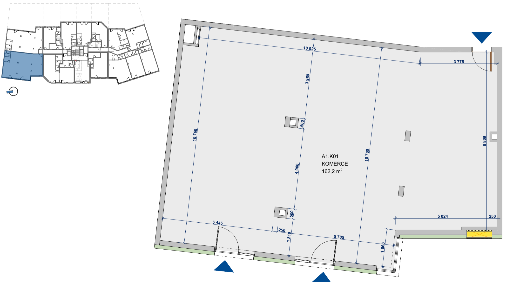
SCHÉMA PODLAŽÍ
