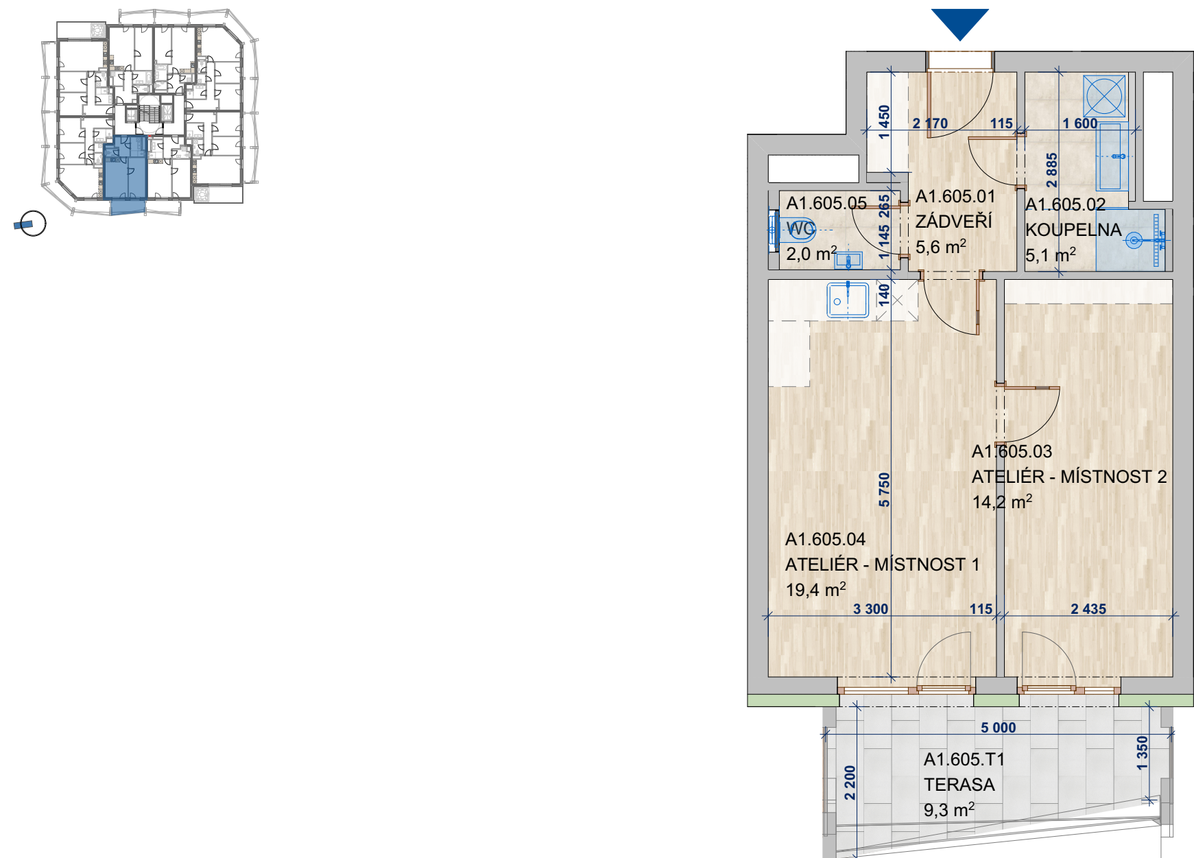
SCHÉMA PODLAŽÍ
