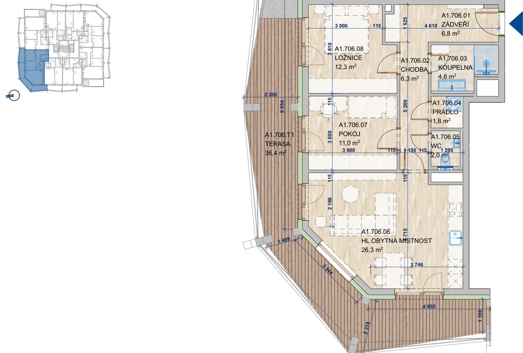
SCHÉMA PODLAŽÍ
