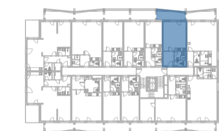
SCHÉMA PODLAŽÍ
