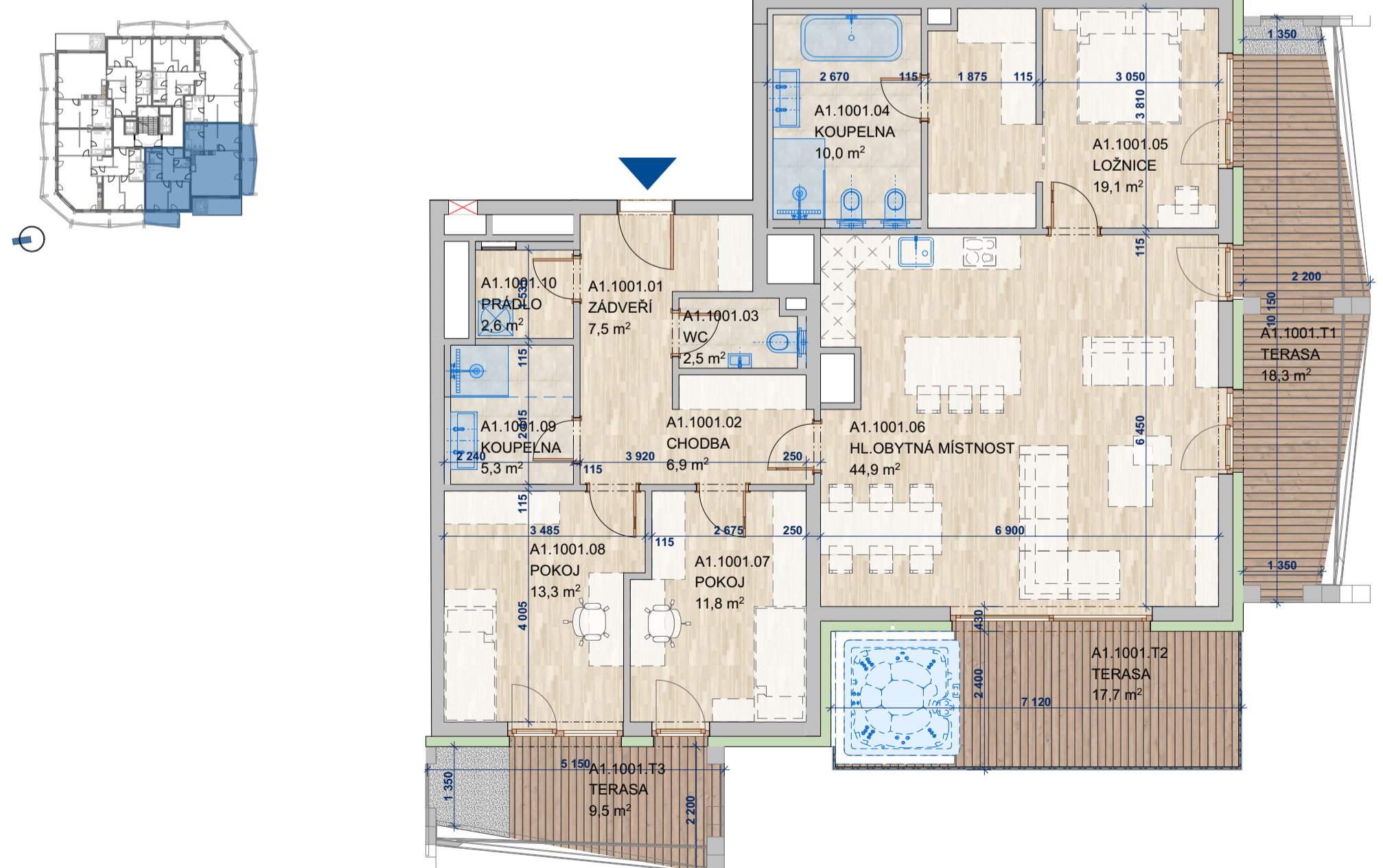
SCHÉMA PODLAŽÍ
