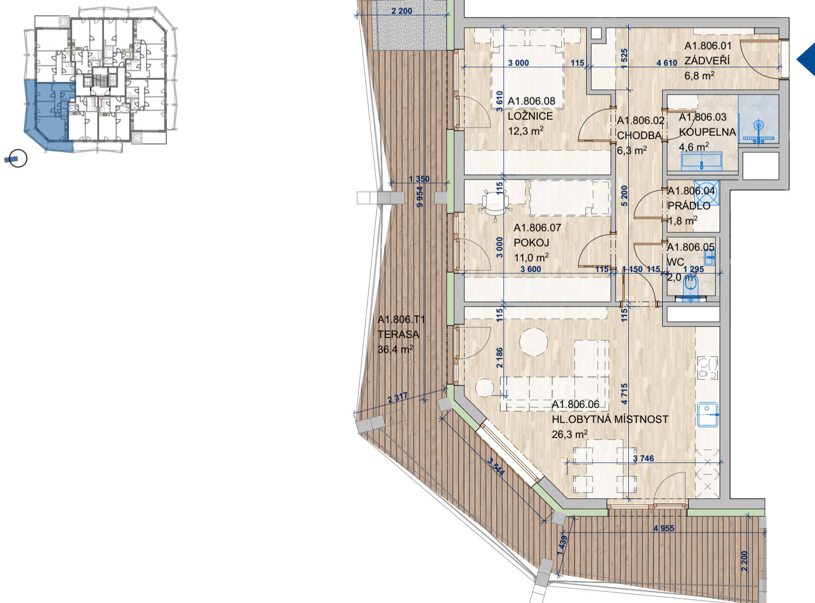
SCHÉMA PODLAŽÍ
