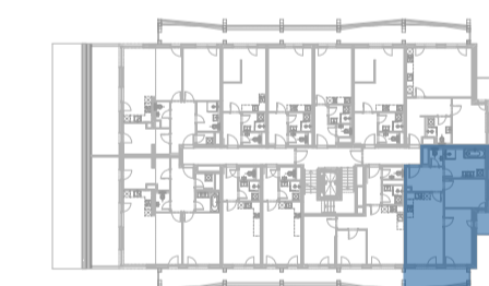
SCHÉMA PODLAŽÍ
