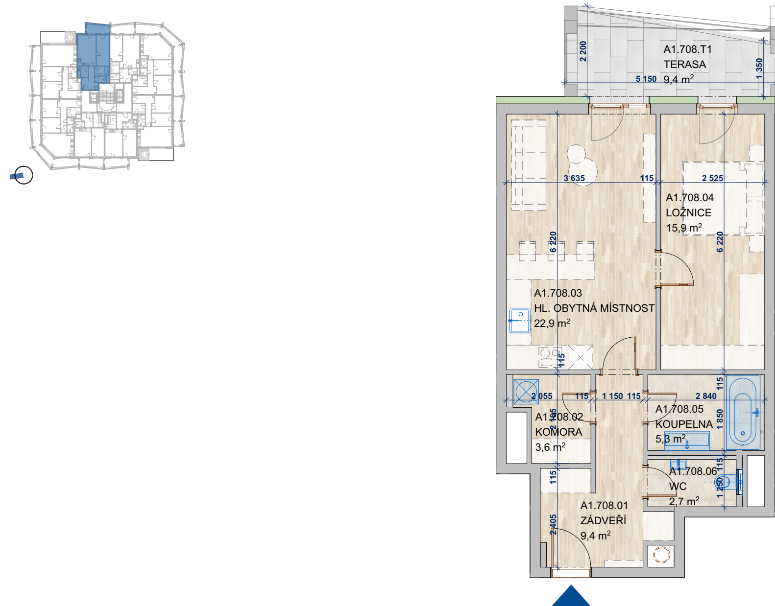
SCHÉMA PODLAŽÍ
