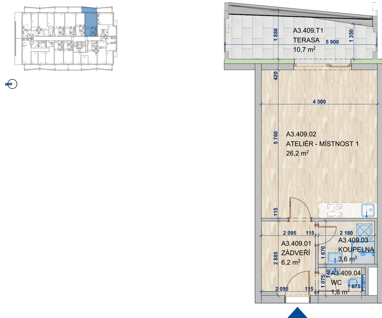
SCHÉMA PODLAŽÍ
