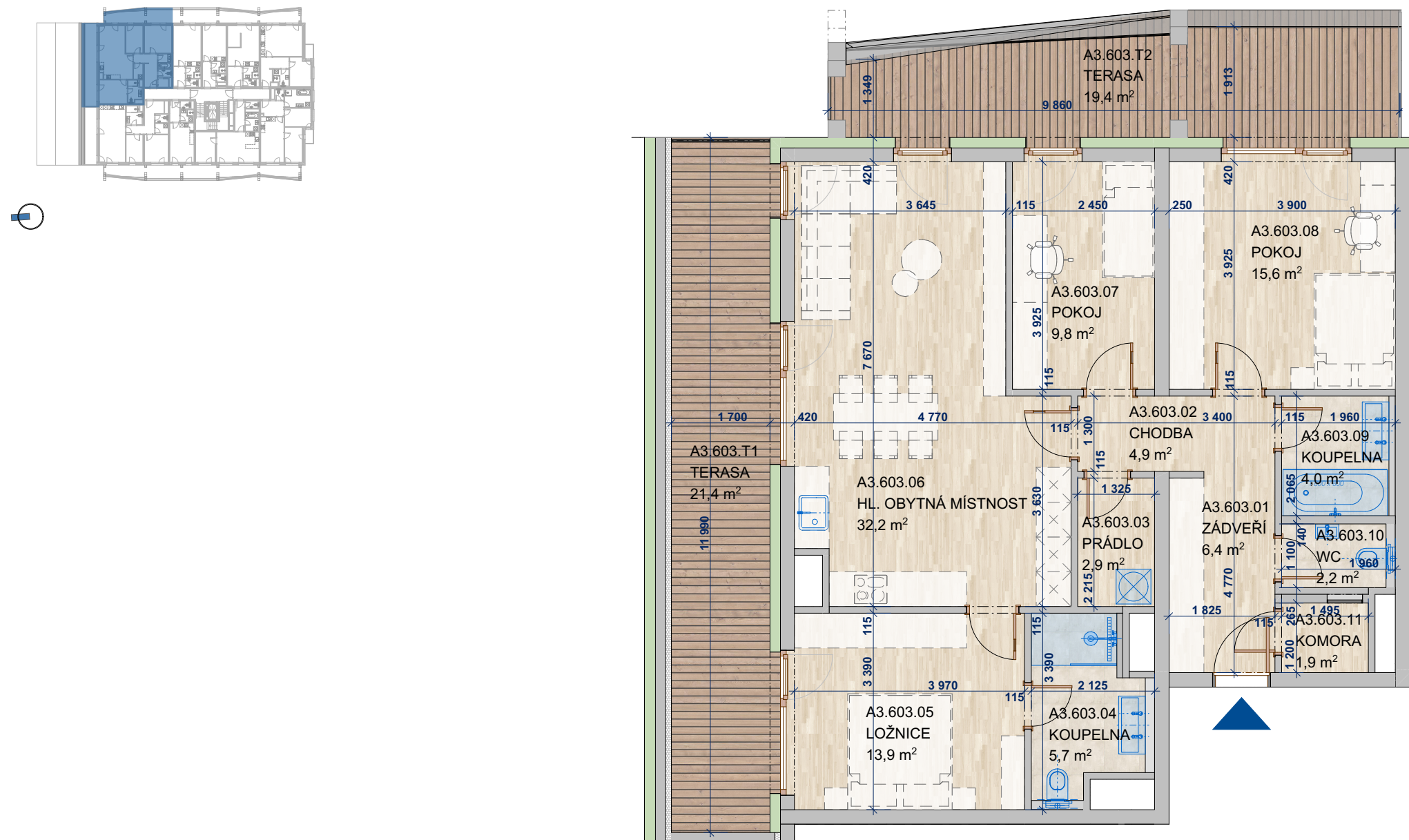
SCHÉMA PODLAŽÍ
