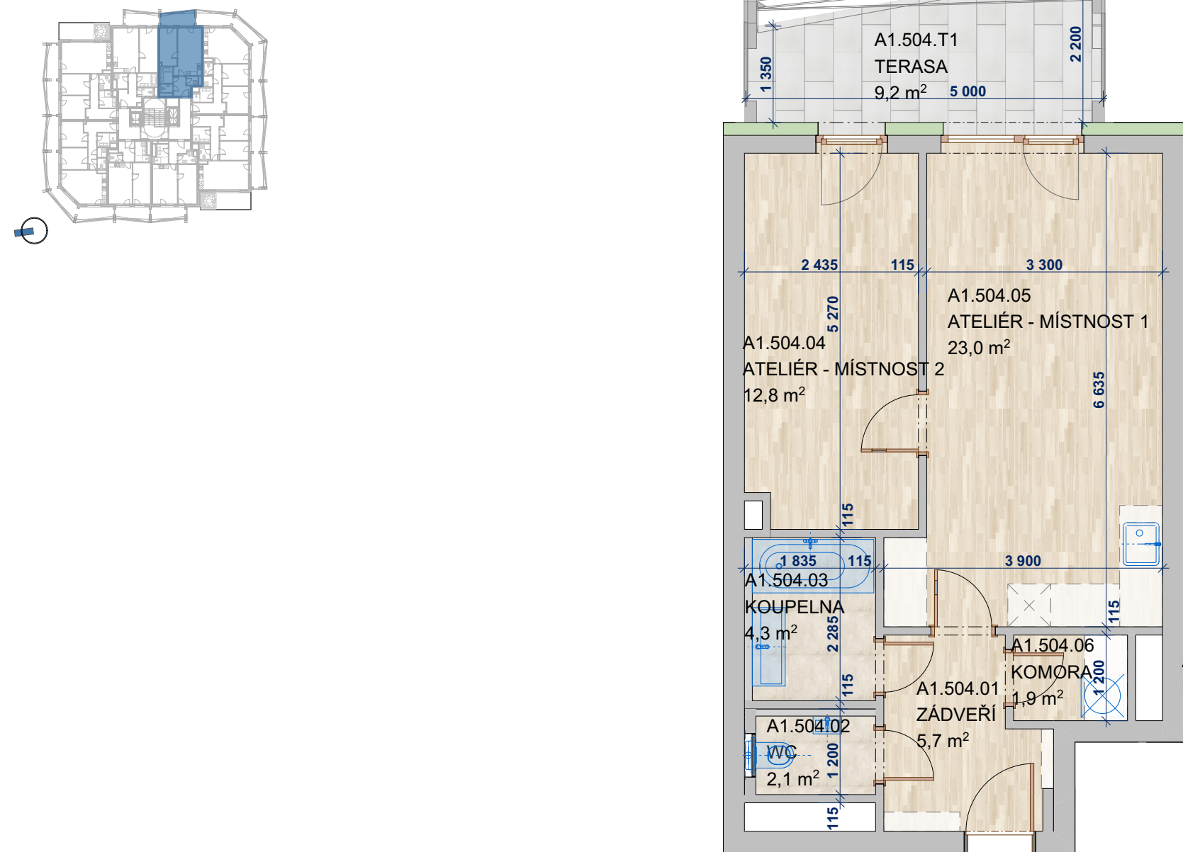
SCHÉMA PODLAŽÍ
