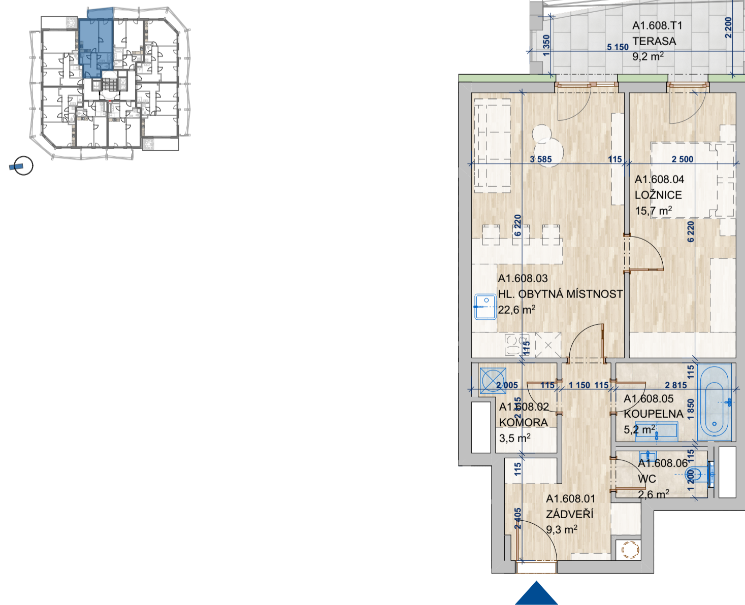
SCHÉMA PODLAŽÍ
